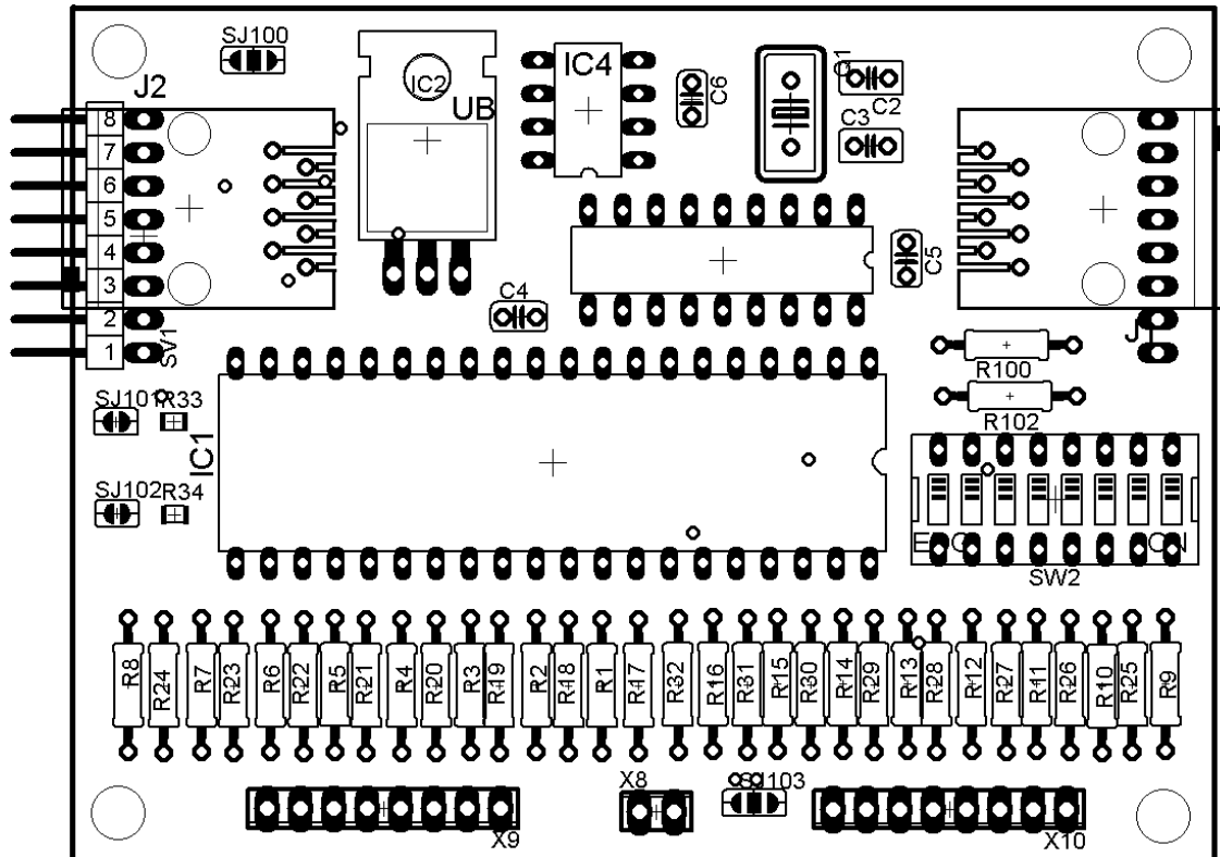
Stückliste zum SwitchPad
